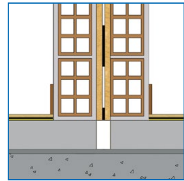
Encuentro de divisoria sobre mortero
