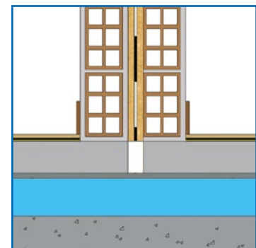
Encuentro de divisoria sobre mortero
