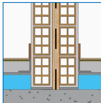
Encuentro de divisoria sobre banda
