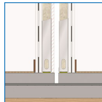
Encuentro de forjado con divisoria (parte inferior)
