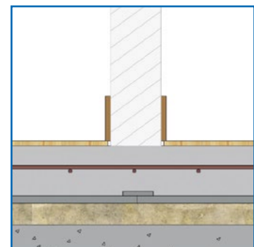
Encuentro con tabiquería interior
