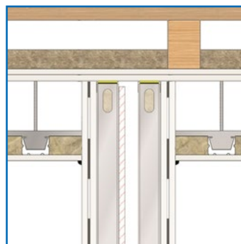
Encuentro de forjado con divisoria (parte superior)
