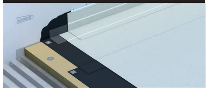
SISTEMA NOX2
