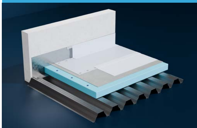
SISTEMA NTV16
