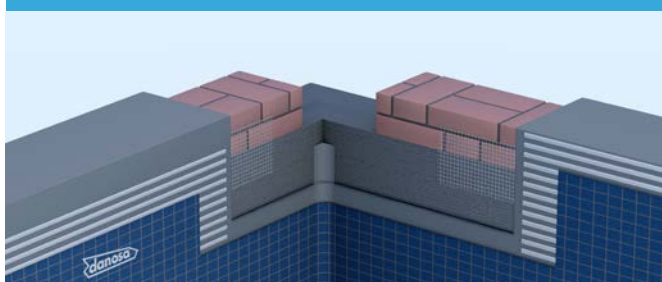
SISTEMA PFE8
