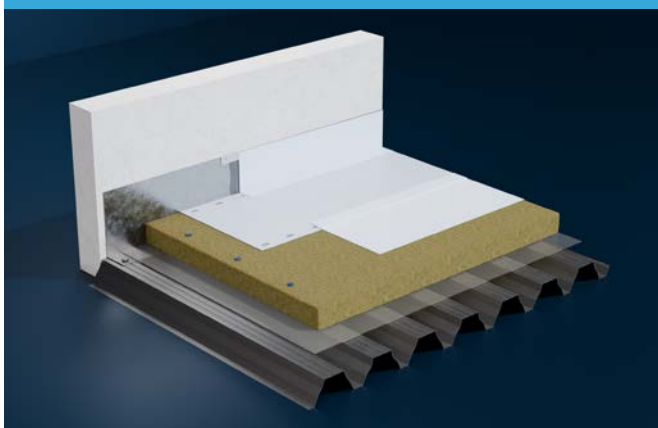
SISTEMA NTV15
