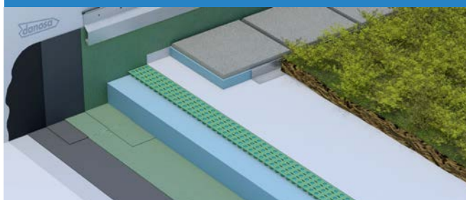
SYSTÈME TVI1
