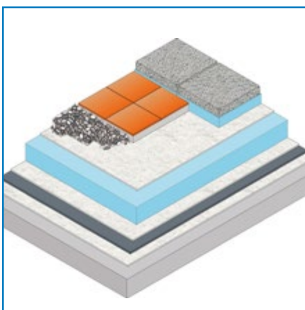
Coberturas lastradas
