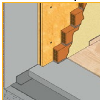
Sistema de pavimento flutuante em estabelecimentos
