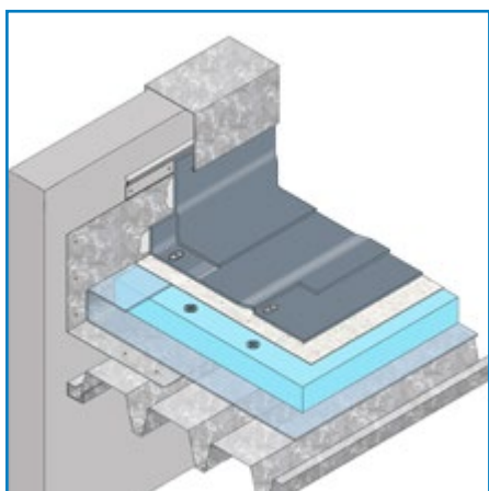
Coberturas planas fixadas mecanicamente
