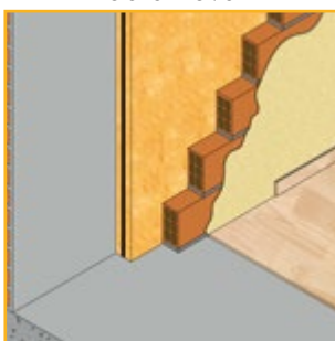
Alvenaria tradicional em reabilitação
