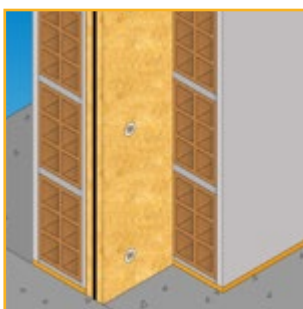
Alvenaria tradicional em obra nova
