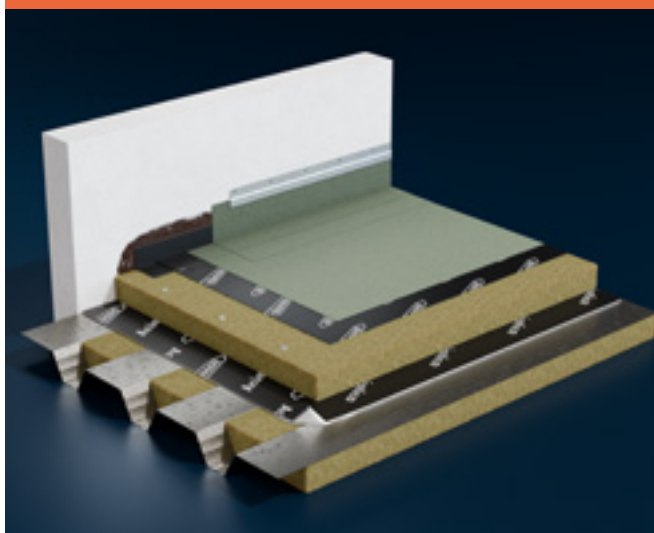
COBERTURA DECK ACÚSTICA COM MEMBRANA BETUMINOSA
